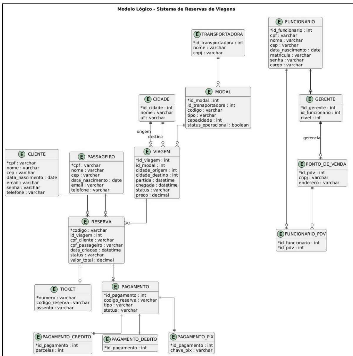
Figura 3.5.1 - Diagrama de Entidade-Relacionamento Lógico
