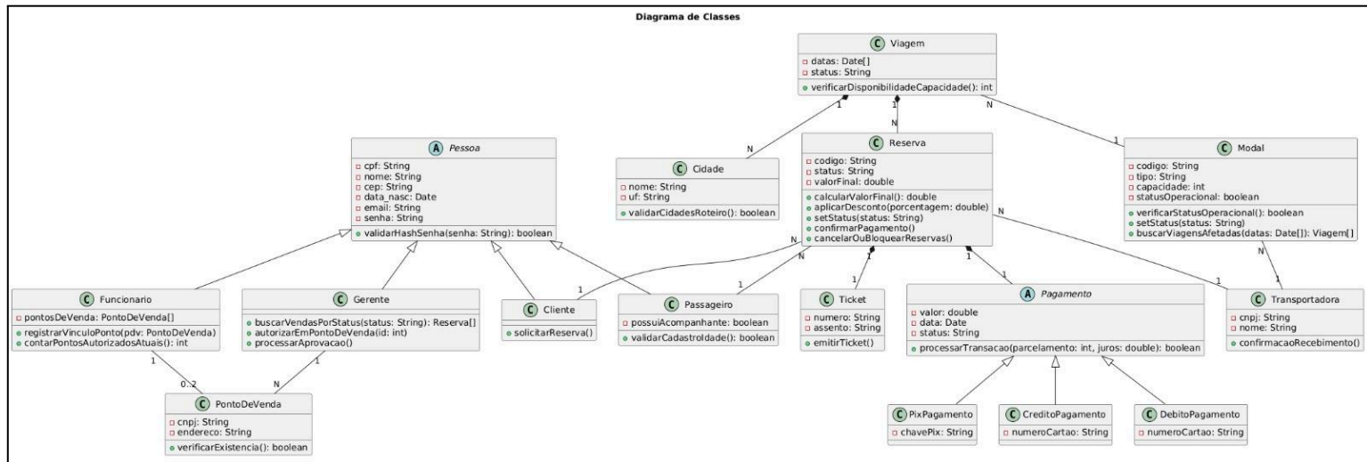
Figura 3.2 - Diagrama de Classes
